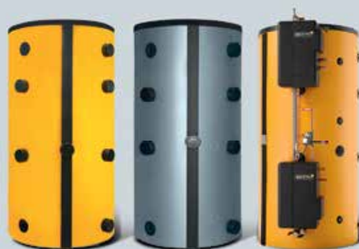
Buffer de estratificación ETA SP y SPS (600, 825, 1.000, 1.100, 1.650 y 2.200 litros) con Módulos de Agua Caliente Sanitaria y Carga Solar
